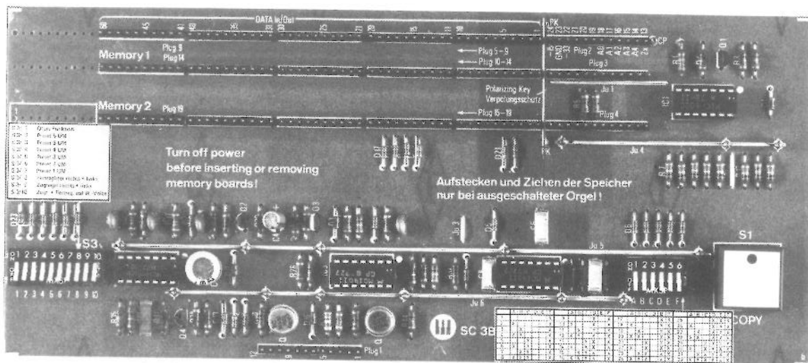
Abb. 3: Die Speichergrundplatte für das Untermanual (fertig bestückte Platine SC 3 B)
