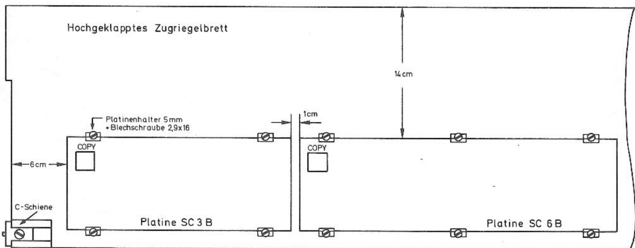
Abb. 31: Einbau der Speichergrundplatten unter dem Zugriegelbrett
