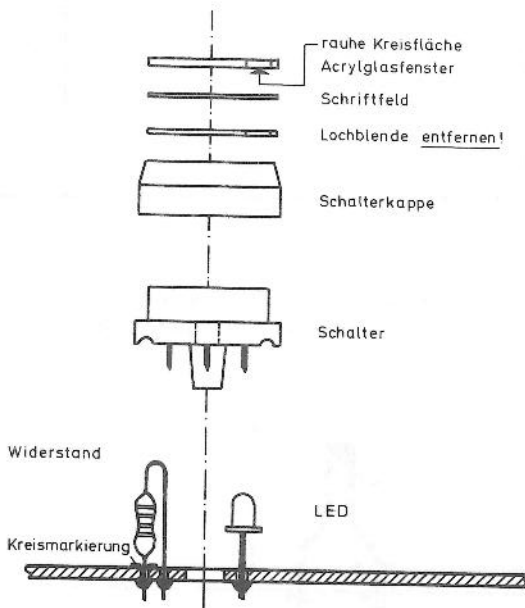
Abb. 17: Einbau der Taster und Schalter
