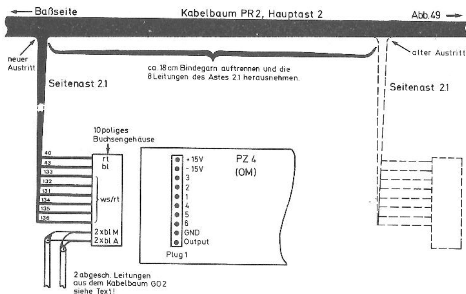
Abb. 48: Änderung des Kabelbaums PR 2 am Ast 2.1 (gilt auch für den Ast 2.2)
