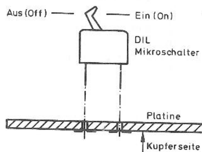
Abb. 13: Einbau eines DIL-Mikroschalters (Seitenansicht)
