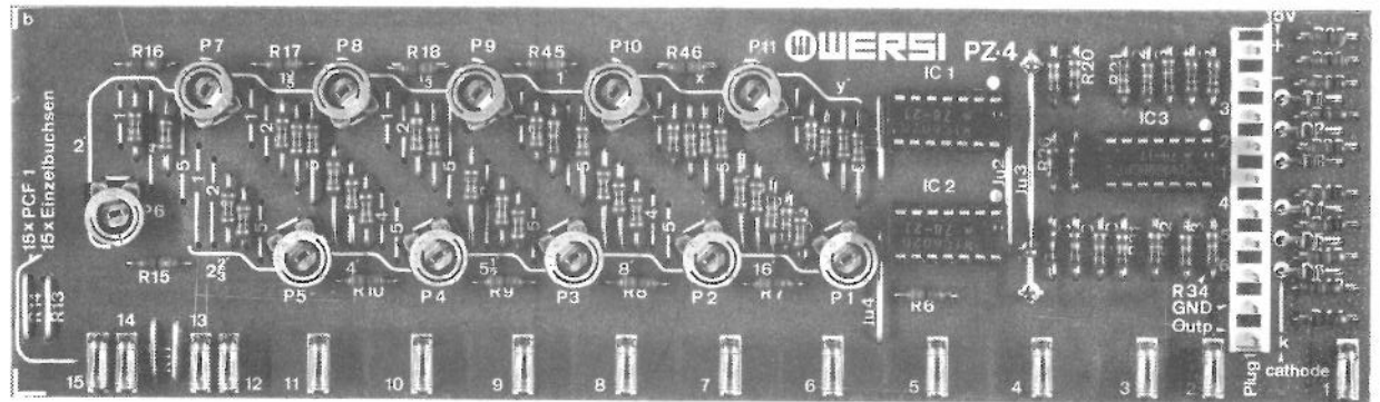
Abb. 22: Fertig bestückte Platine PZ 4
