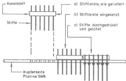
Abb. 29: Einsetzen der Mini-Stiftleisten in die Platine SW 8
