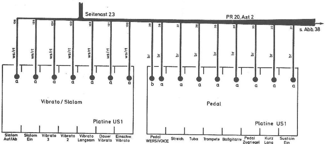
Abb. 39: Ast 2 an den Schaltergruppen Pedal und Vibrato/Slalom
