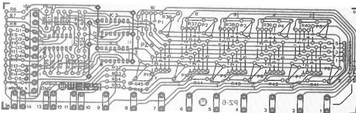
Abb. 23: Positionsdruck und Leiterbahnen der Platine PZ 6
