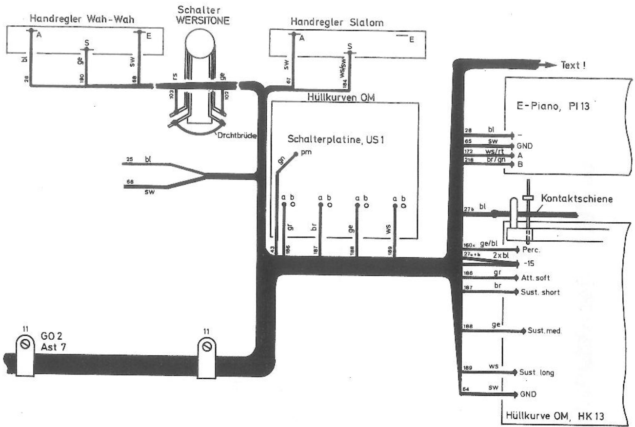
Abb. 44: Der Kabelbaum GO 2 vor der Änderung
