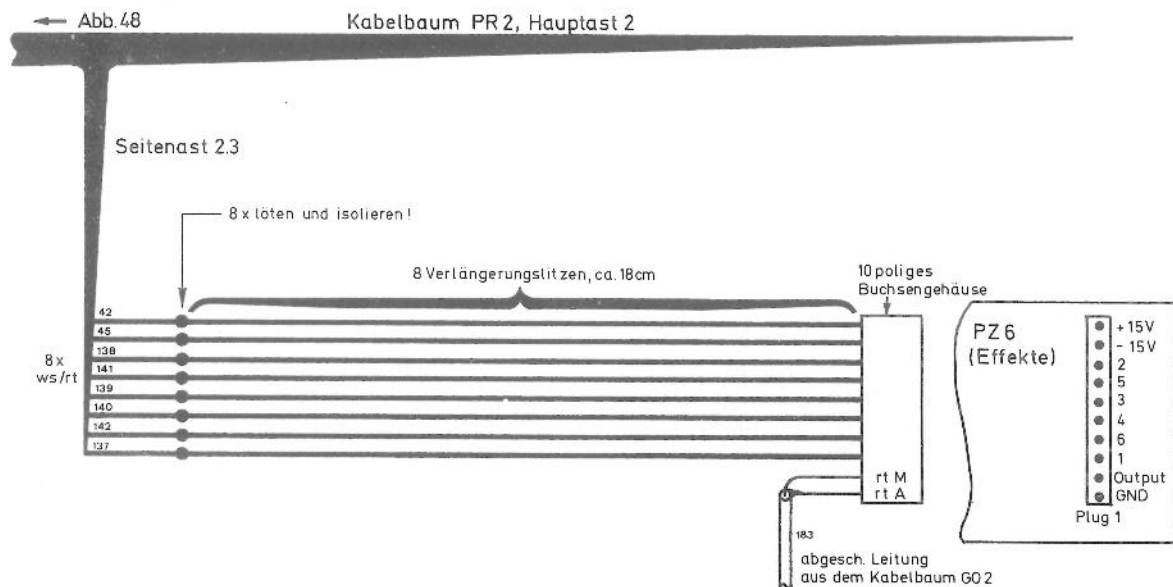
Abb. 49: Änderung des Kabelbaums PR 2 am Ast 2.3
