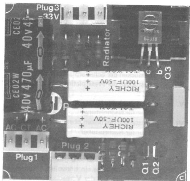
Abb. 9: Fertig bestücktes Zusatznetzteil PS 6
