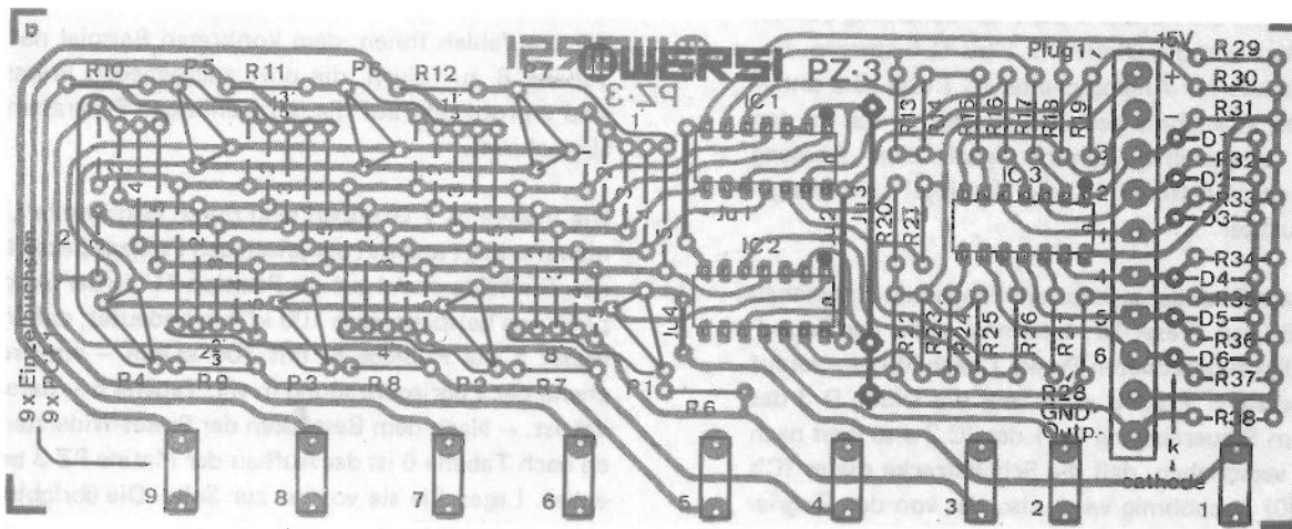
Abb. 19: Positionsdruck und Leiterbahnen der Platine PZ 3
