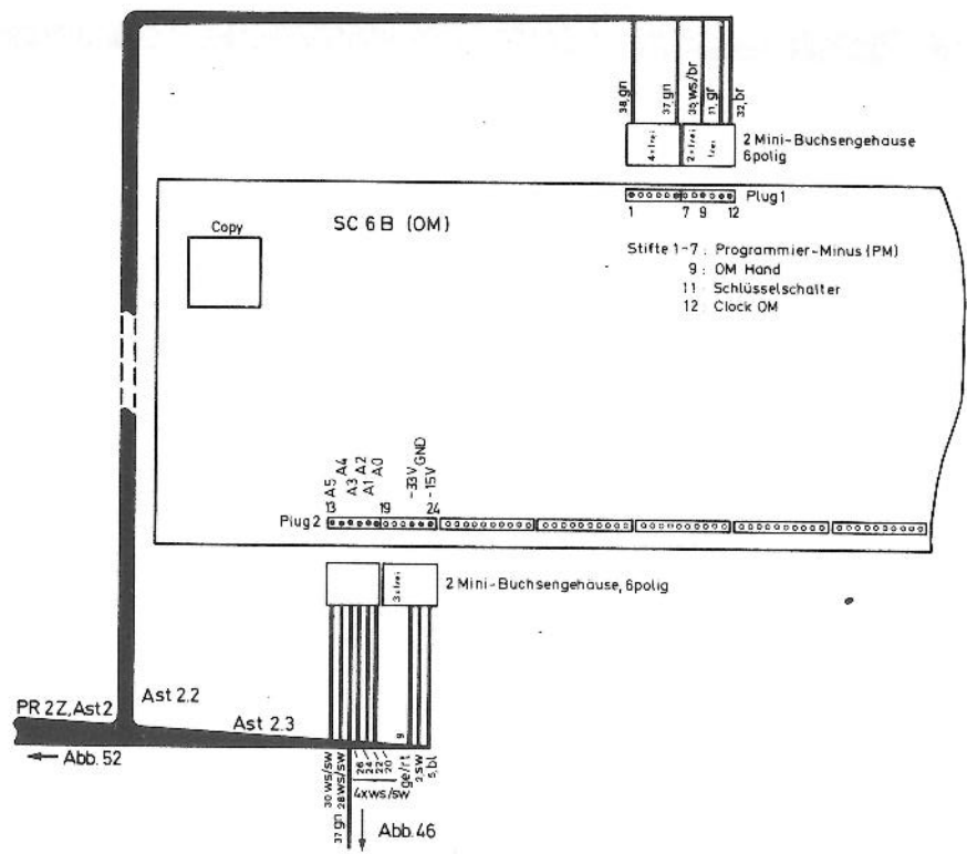
Abb. 53: Der Zusatzkabelbaum PR 2 Z an der Platine SC 6 B
