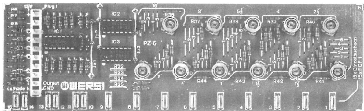
Abb. 24: Fertig bestückte Platine PZ 6
